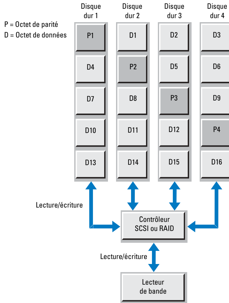
Figure 1-4. Exemple de configuration RAID 5
